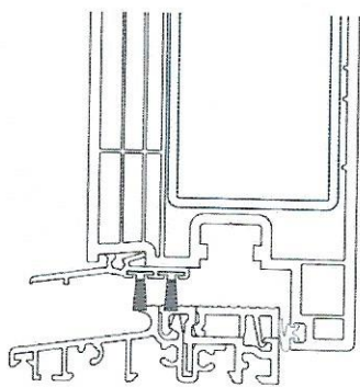
Apertura all'interno
