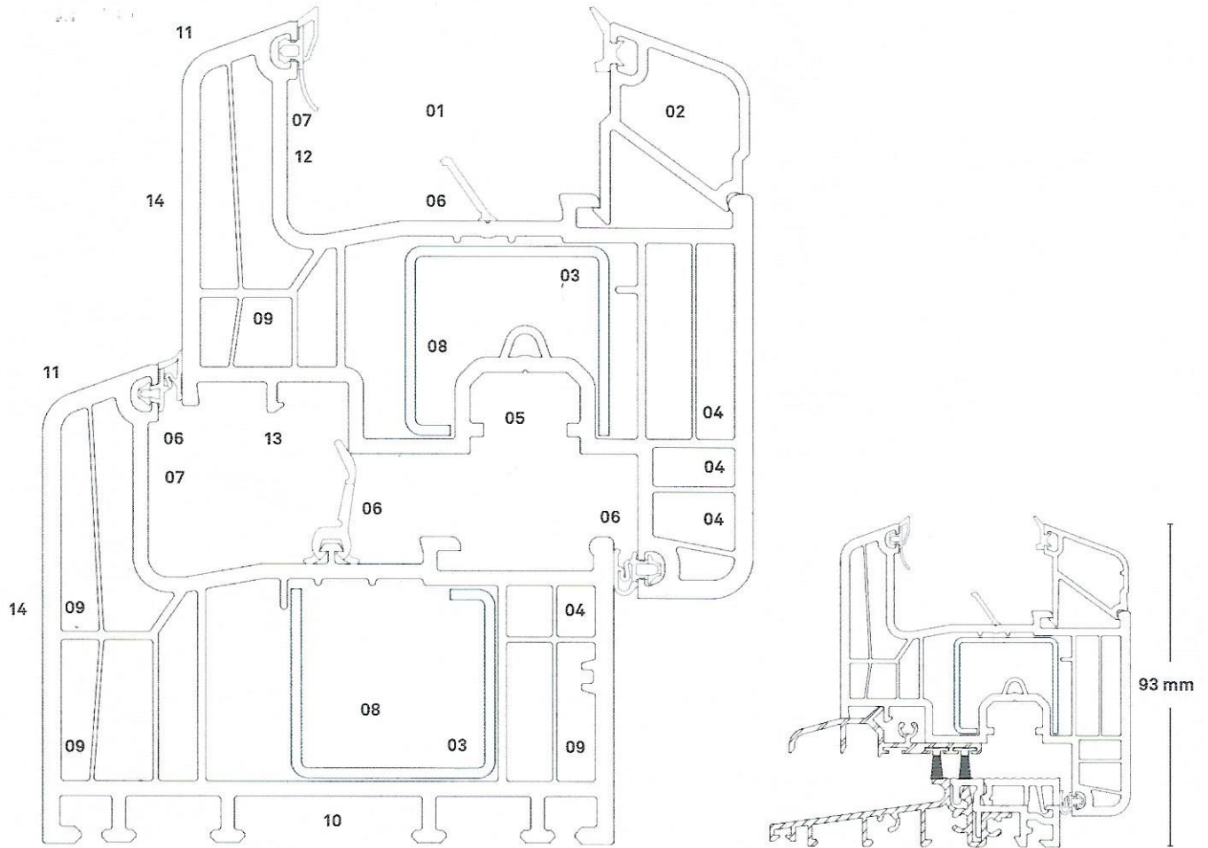
Fig. 1:2 La nuova soglia piatta per porte balcone
